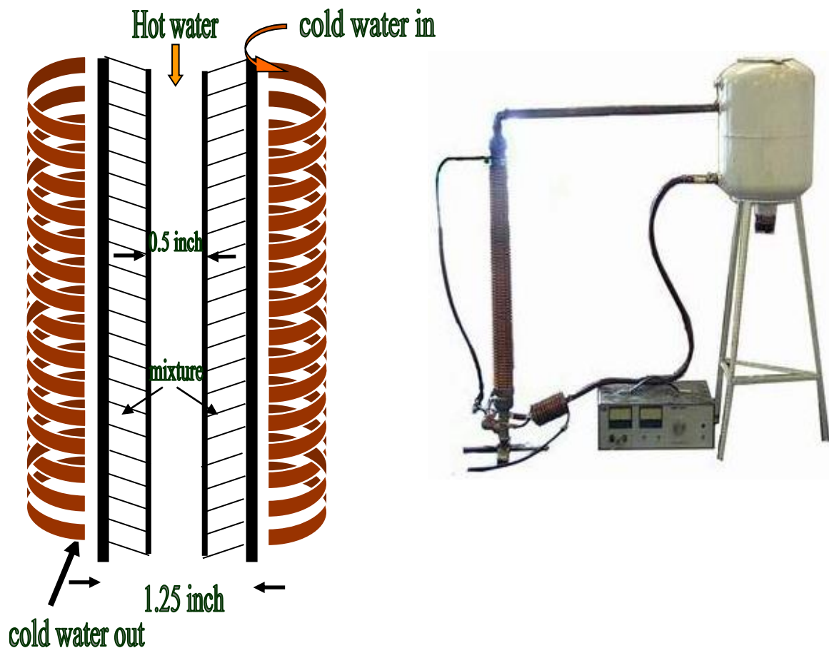
Fig. (1-a) Experimental Apparatus
