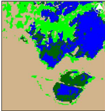
شكل (3) يوضح التصنيف الموجه للغطاء الأرضي لصورة القمر الصناعي Landsat لهور الكرماشية لغطاء الأرضي لصورة القمر
