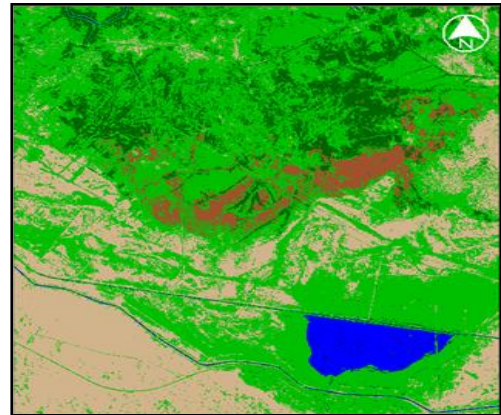
شكل (3) يوضح التصنيف الموجه للغطاء الأرضي لصورة القمر الصناعي Landsat لهور الكرماشية لغطاء الأرضي لصورة القمر
