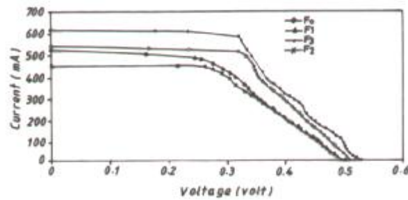
شكل (3) خصائص التيار-فولتية للمركز الحوضي ثنائي المرايا وعنسات فرنيل المختلفة و بدون تبريد
