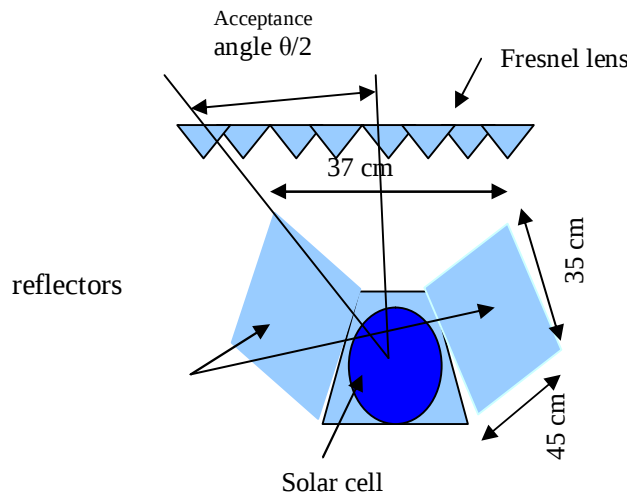
شكل (1) المركز الحوضي المركب مع عدسات فرينل
