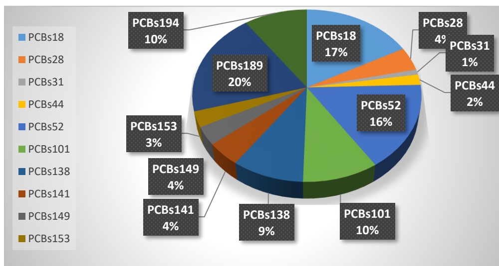
شكل (2): النسبة المئوية لمركبات PCBs في المياه
