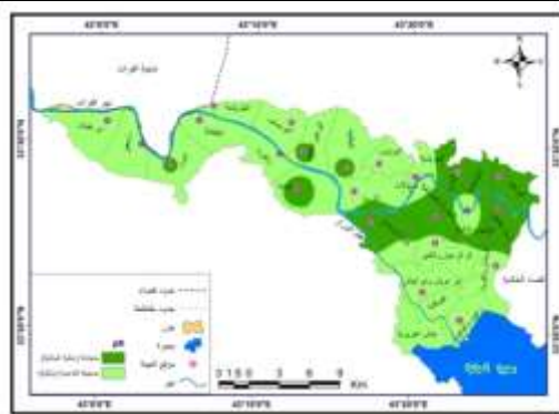
خريطة (٥) : صلاحية التربة بالنسبة الى المادة العضوية
