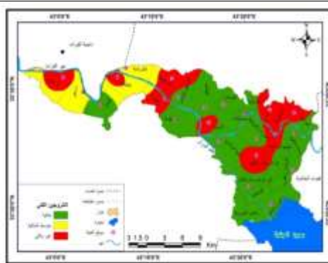
خريطة (١١) : تصنيف النتروجين الكلي في التربة
