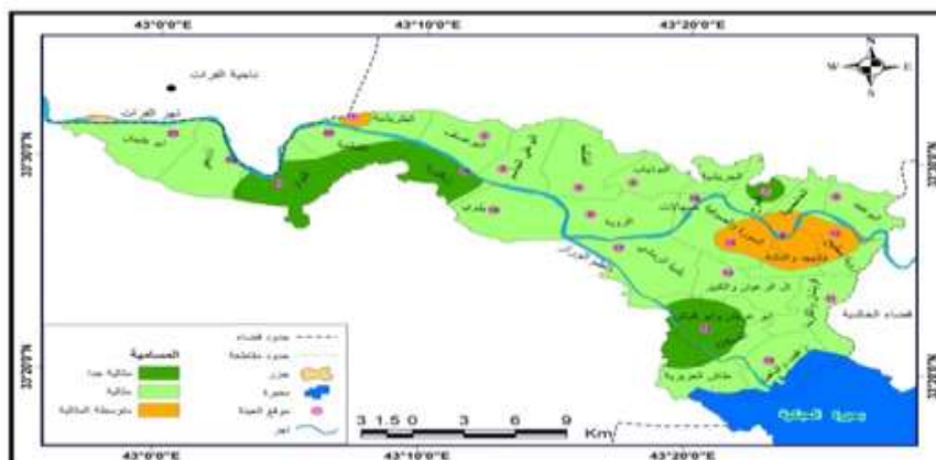
خريطة (٤) : تصنيف التربة بحسب النسبة المئوية لحجم المسامات.
