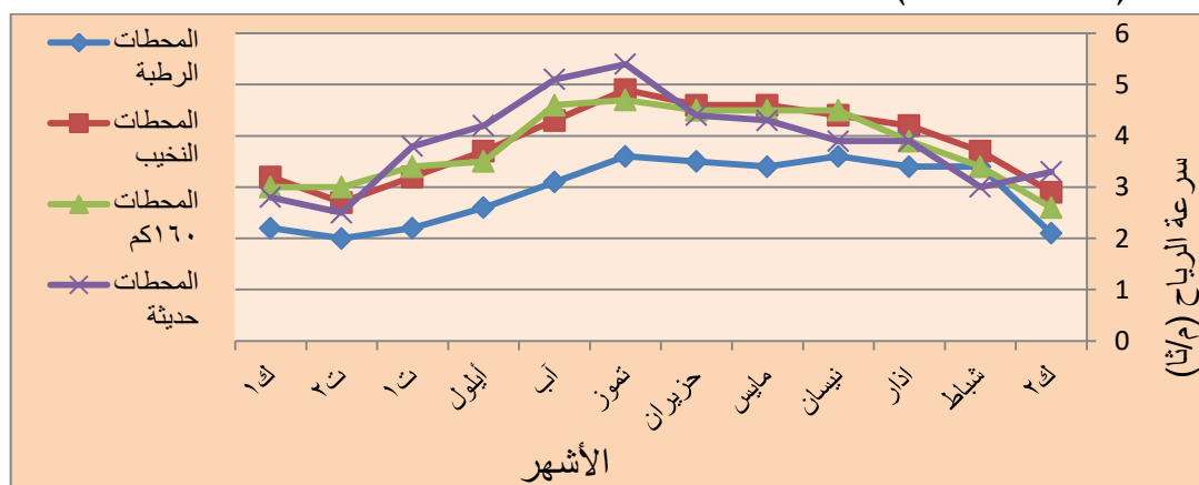
شكل (٣) المعدلات الشهرية لسرعة الرياح (م/ثا) لمحطات (الرطبة، النخيب، 160 كم، حديثة) للمدة (1988-2018)
