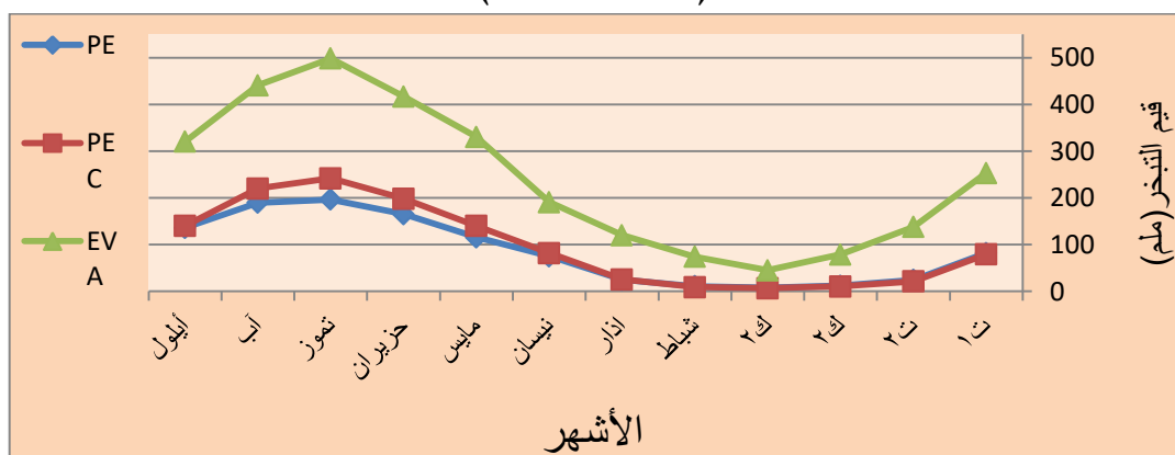
شكل (٨) قيم التبخر النتج الكامن والمصحح (ملم) بحسب ثورنثويت لمحطة 160 للمدة (2018-1988)
