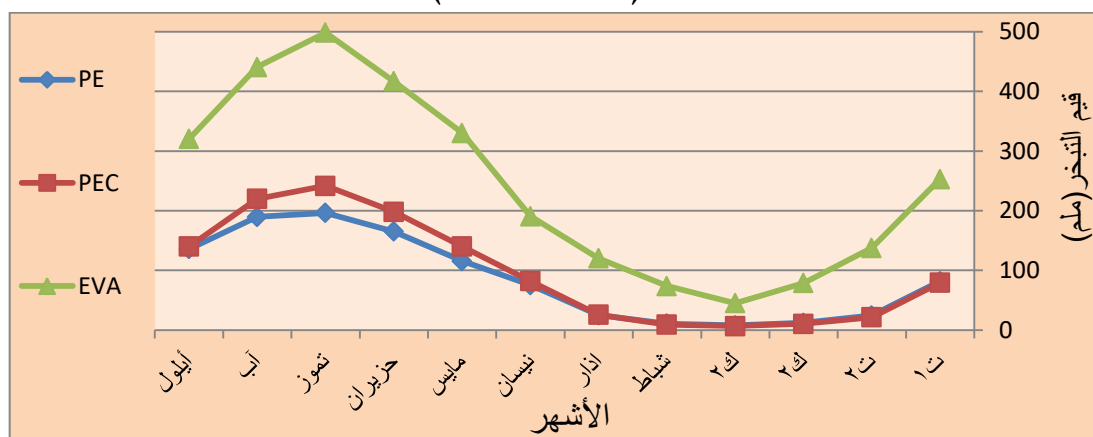
شكل (٦) قيم التبخر النتج الكامن والمصحح (ملم) بحسب ثورنثويت لمحطة الرطبة للمدة (1988-2018)
