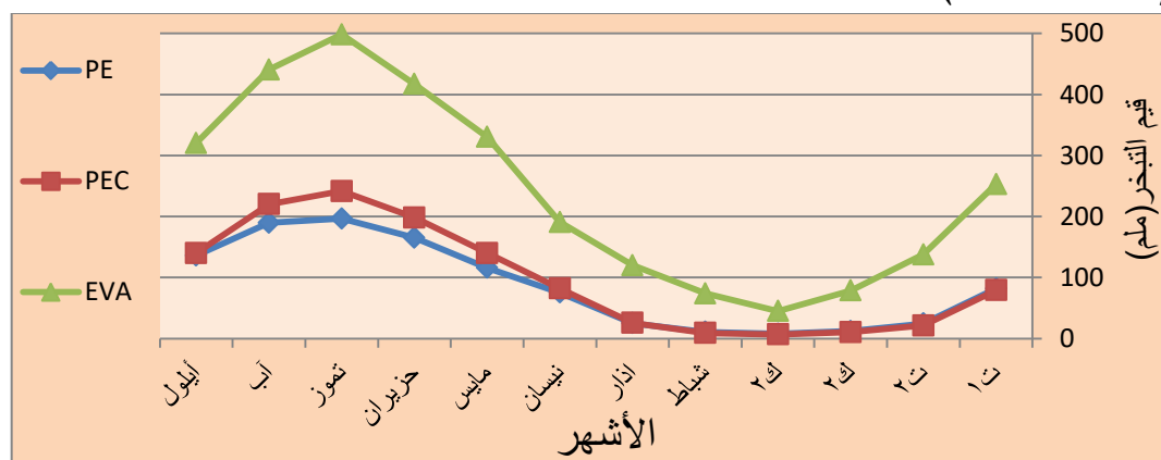
شكل (٧) قيم التبخر النتج الكامن والمصحح (ملم) بحسب ثورنثويت لمحطة النخيب للمدة (1988-2018)
