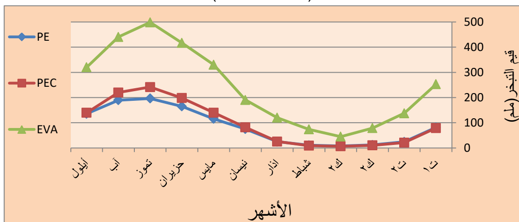
شكل (٩) قيم التبخر النتج الكامن والمصحح (ملم) بحسب ثورنثويت لمحطة حديثة للمدة (2018-1988)
