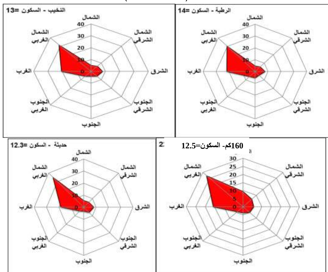
شكل (٤) النسبة المئوية لتكرار اتجاهات الرياح لمحطات (الرطبة، النخيب، 160 كم، حديثة للمدة (1988-2018)
