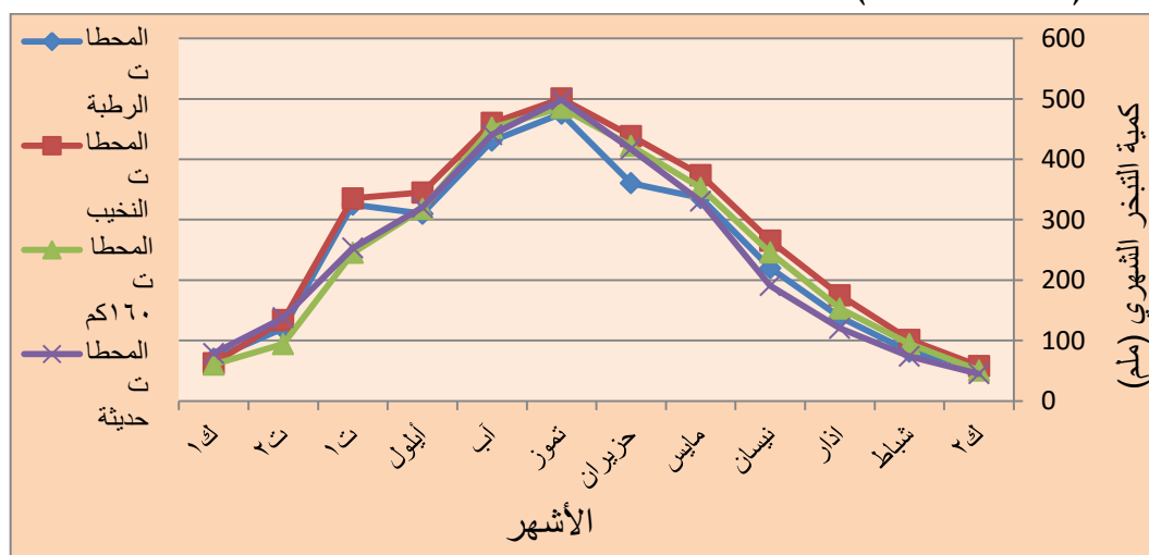
شكل (٥) معدل كمية التبخر الشهري (ملم) لمحطات (الرطبة، النخيب، 160 كم، حديثة) للمدة (1988-2018)
