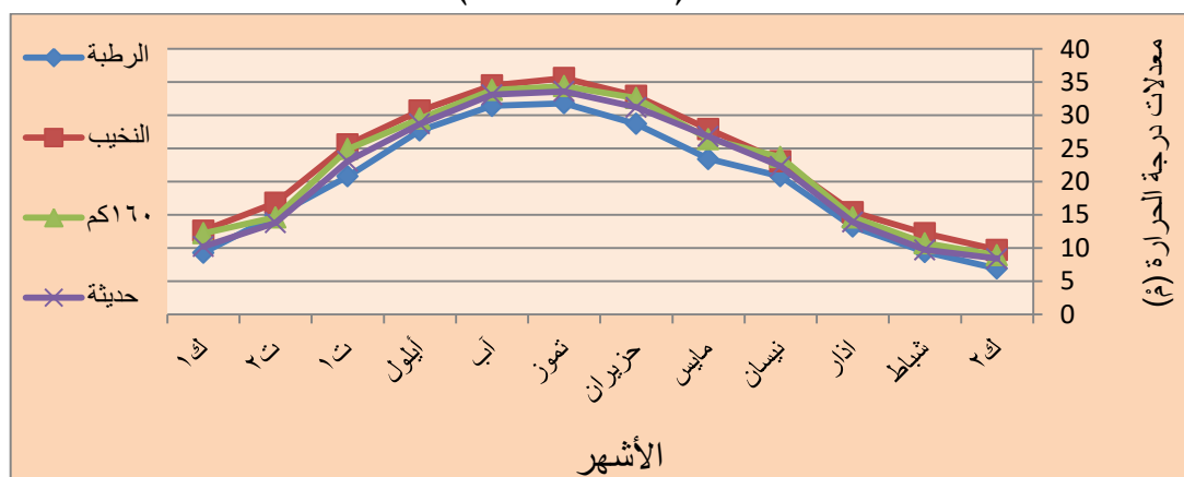
شكل (١) معدلات درجة الحرارة (م) لمحطات (الرطبة، النخيب، ١٦٠ كم، حديثة) للمدة (1988-2018)
