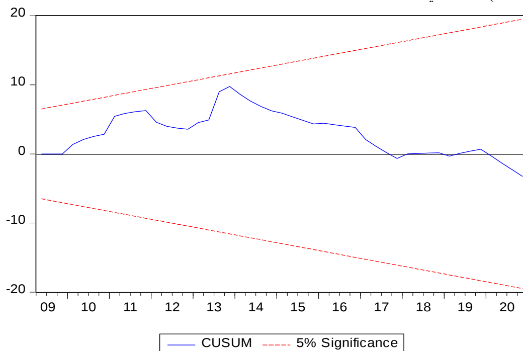
الشكل (٢): اختبار المجموع التراكمي للبواقي Cusum
