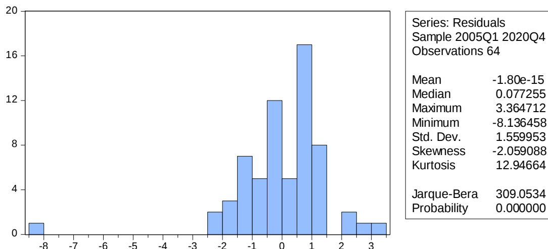
الشكل (١): التوزيع الطبيعي لبواقي نموذج
