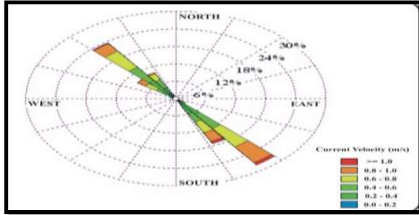
الشكل (٧) سرعة واتجاه التيارات البحرية في خور عبدالله. عن (Al-Hasem, 2018)
