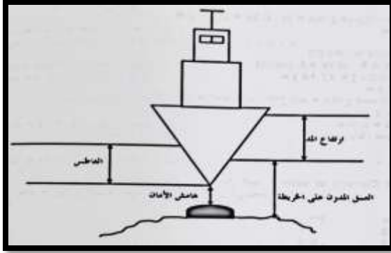
الشكل (٣) تحقق المرور الامن فوق المناطق الضحلة.
