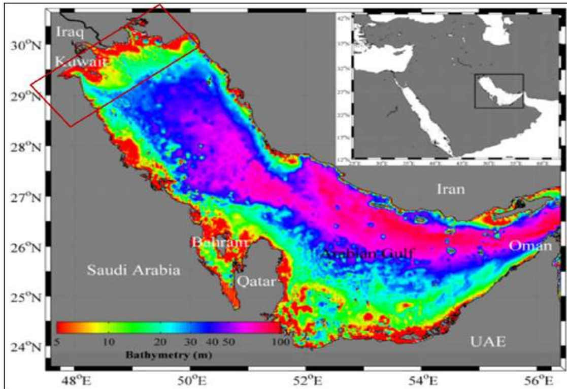
الشكل (٦) اعماق الخليج العربي والجهات الساحلية شمال غرب الخليج العربي.
