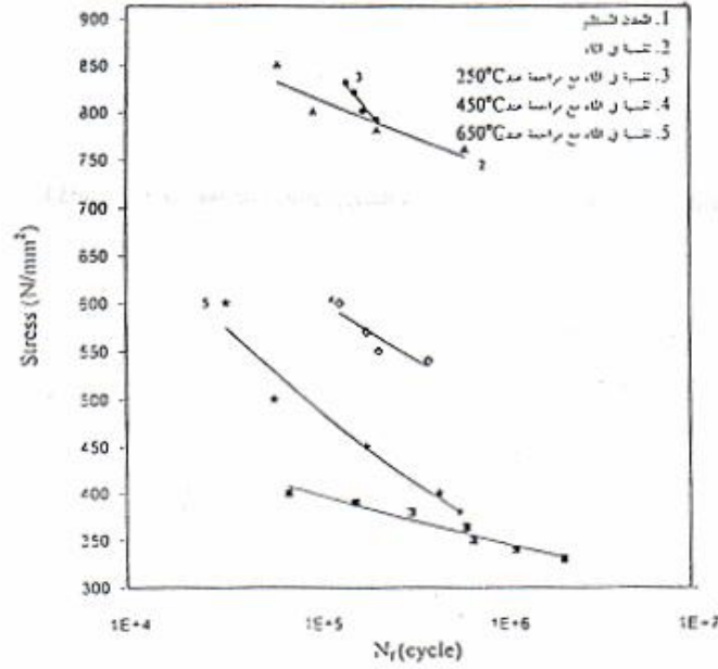
شكل (٦) العلاقة بين الاجهاد - عدد الدورات لفولاذ متوسط الكاربون معامل بطرق مختلفة
