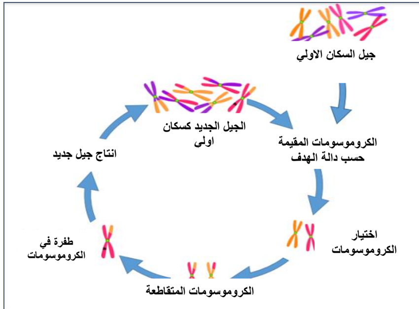
الشكل (٢): يوضح خطوات ومراحل الخوارزمية الجينية
