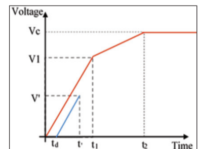
Fig. (8): Four Parameter TRV Envelope [12].
