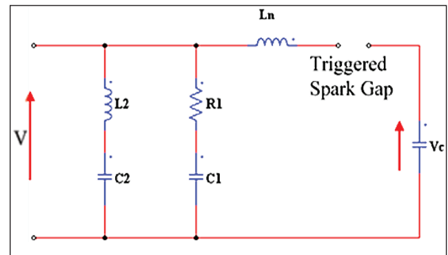
Fig. (7): Four parameters TRV circuit [12].
