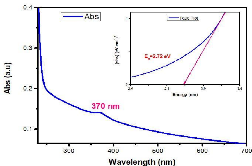
Fig. 4: ZnO NPs UV-Vis spectrum.
