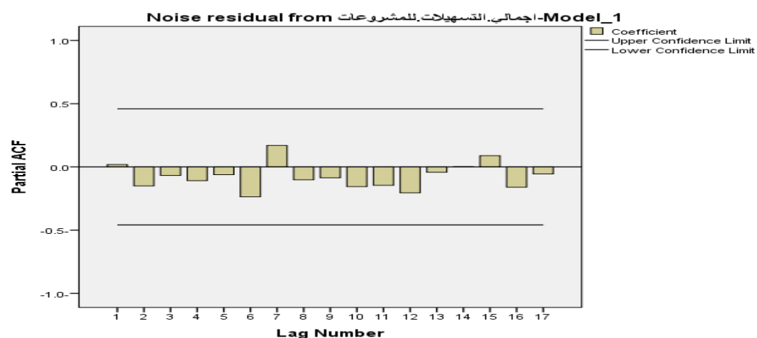
الشكل (٥): دالة الارتباط الذاتي الجزئي للبواقي
