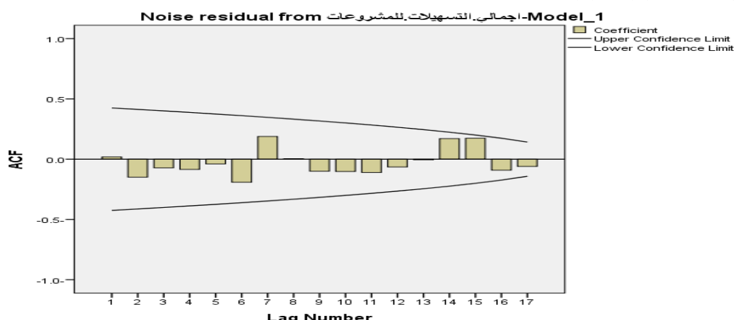
الشكل (٤): دالة الارتباط الذاتي للبواقي
