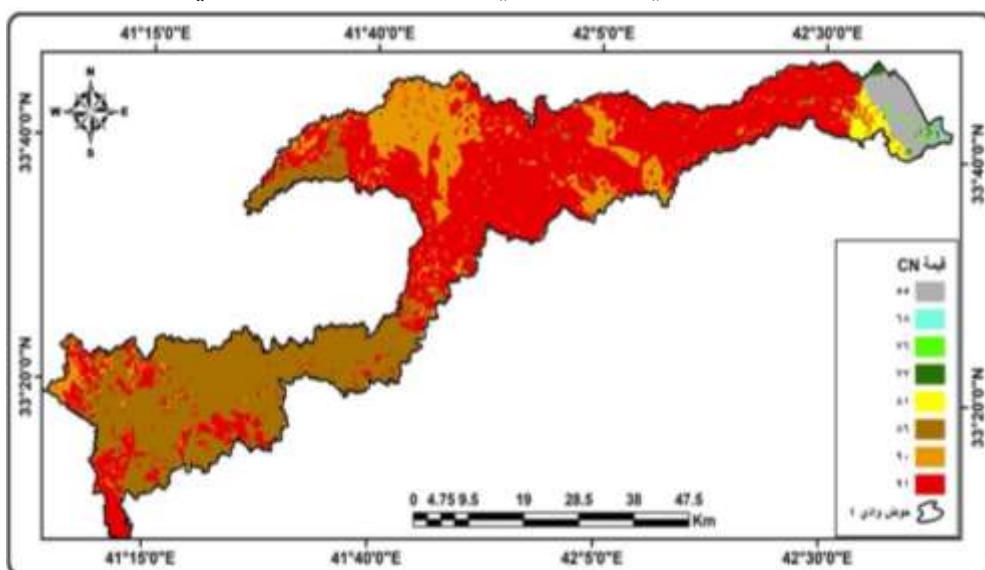
خريطة (٩) توزيع قيم (CN) لحوض وادي (٤)
