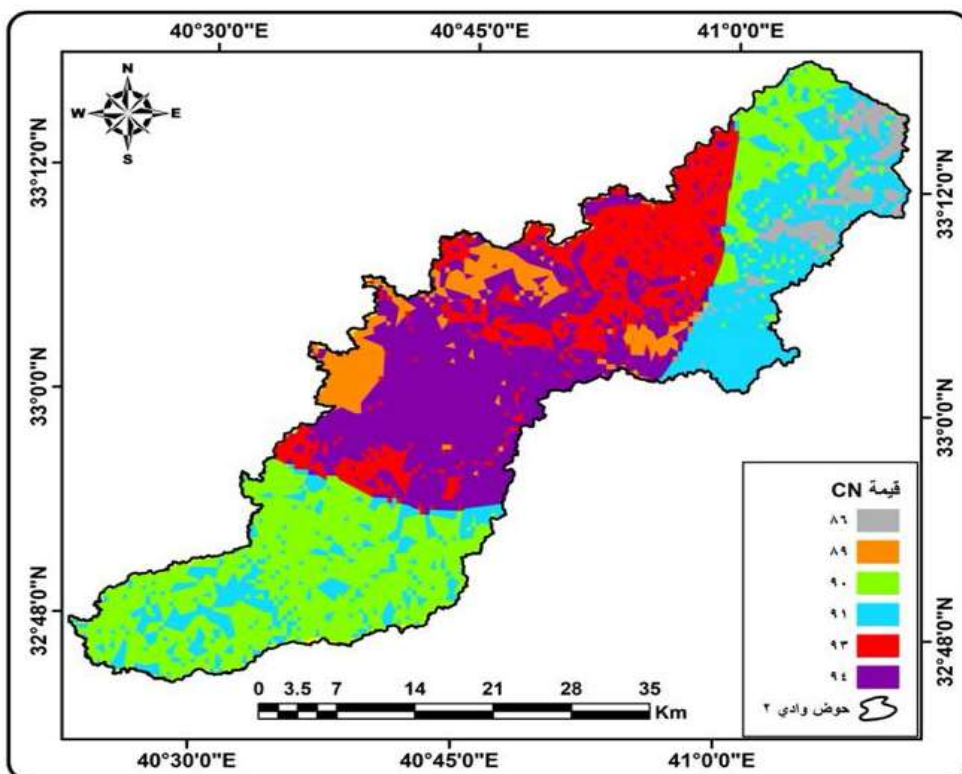
خريطة (7) توزيع قيم (CN) لحوض وادي (٢)
