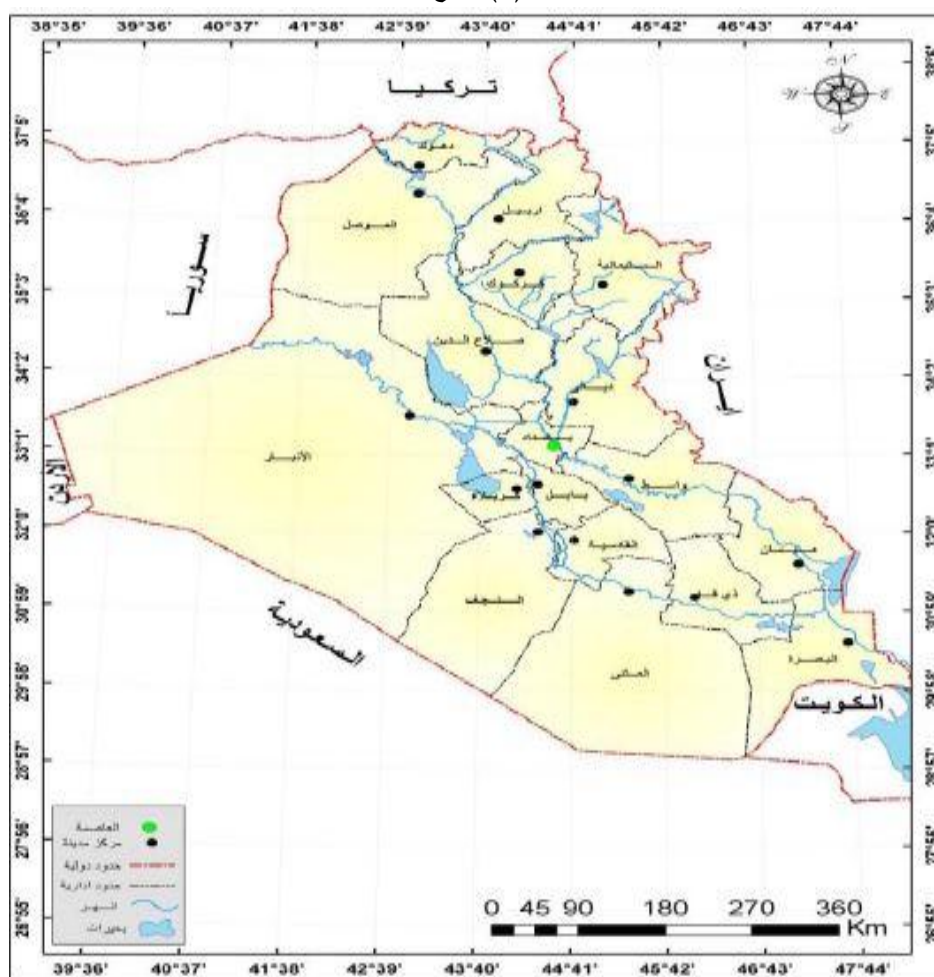
خارطة (1) موقع العراق
