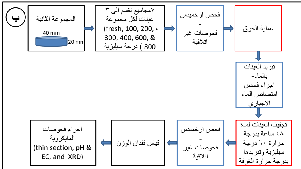
الشكل 6. مخطط المنهج المتبع في الجزء العملي للدراسة الحالية، (أ) نماذج المجموعة الاولى، (ب) نماذج المجموعة الثانية.
