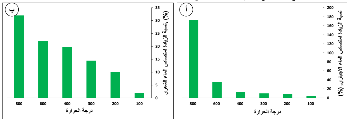
الشكل 10. (أ) التغير في نسب الزيادة في امتصاص الماء الاجباري، (ب) التغير في نسب الزيادة في معامل ارتفاع الماء الشعيري للعينات الصخرية بعد التعرض للحرق.
