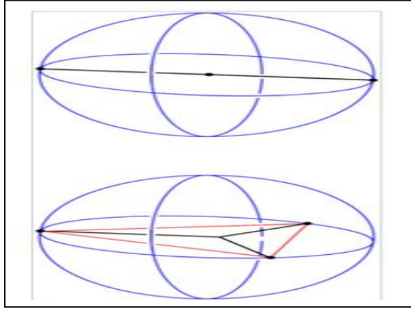
نموذجان من فسيبر لإثنين وثلاثة من أزواج الإلكترونات
