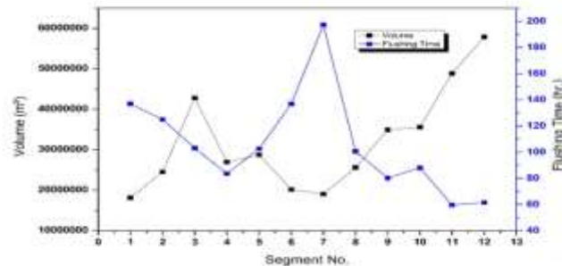
الشكل (9) العلاقة بين زمن التفريغ ( Flushing Time ) ساعة والحجم الكلي ( Volume ) م 3 للقطعة .
