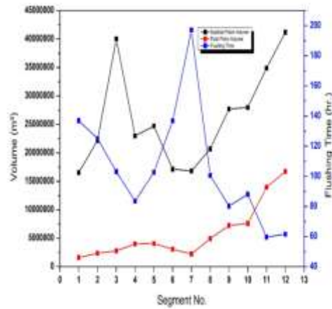
الشكل (9) العلاقة بين زمن التفريغ ( Flushing Time ) ساعة والحجم الكلي ( Volume ) م 3 للقطعة .
