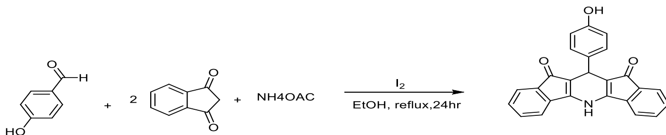
معادلة (1) تحضير المركب IO
