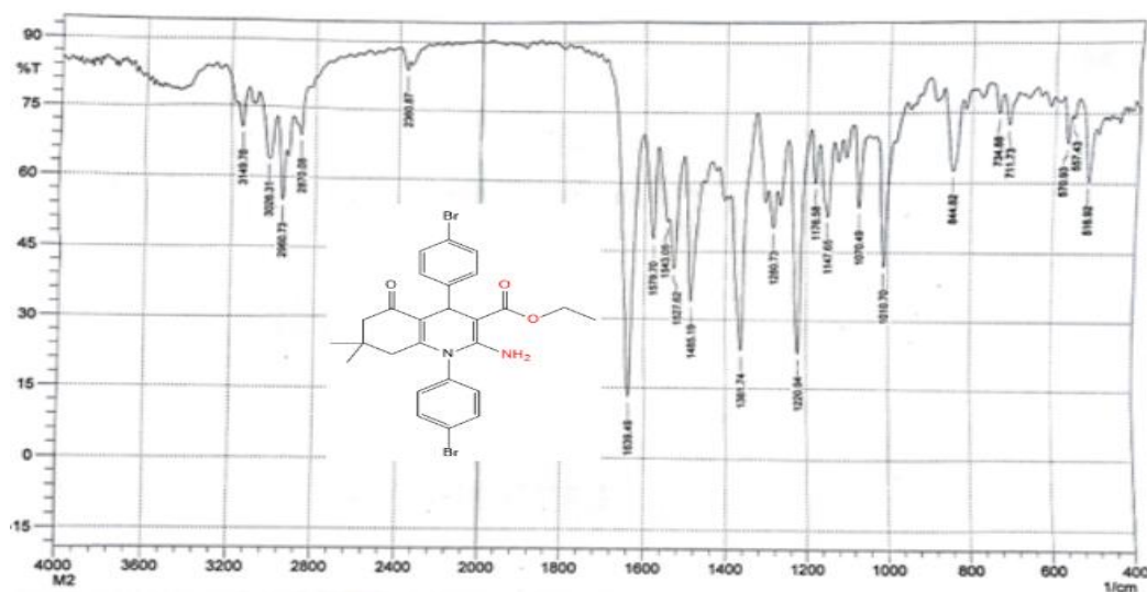
شكل (3.28) طيف IR للمركب Br
