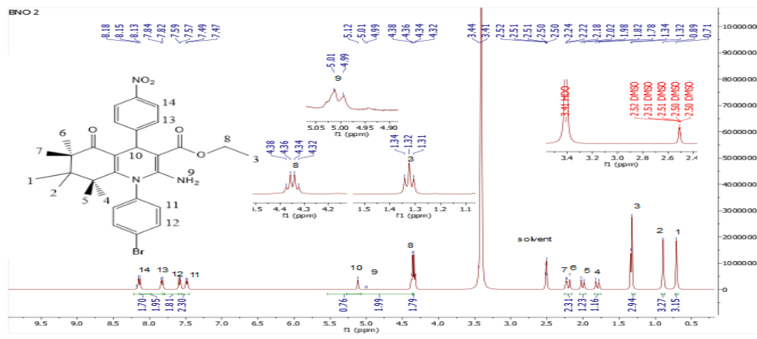
شكل (5) طيف HNMR للمركب BNO2
