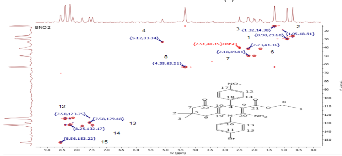
شكل (8) طيف HSCQ للمركب BNO2
