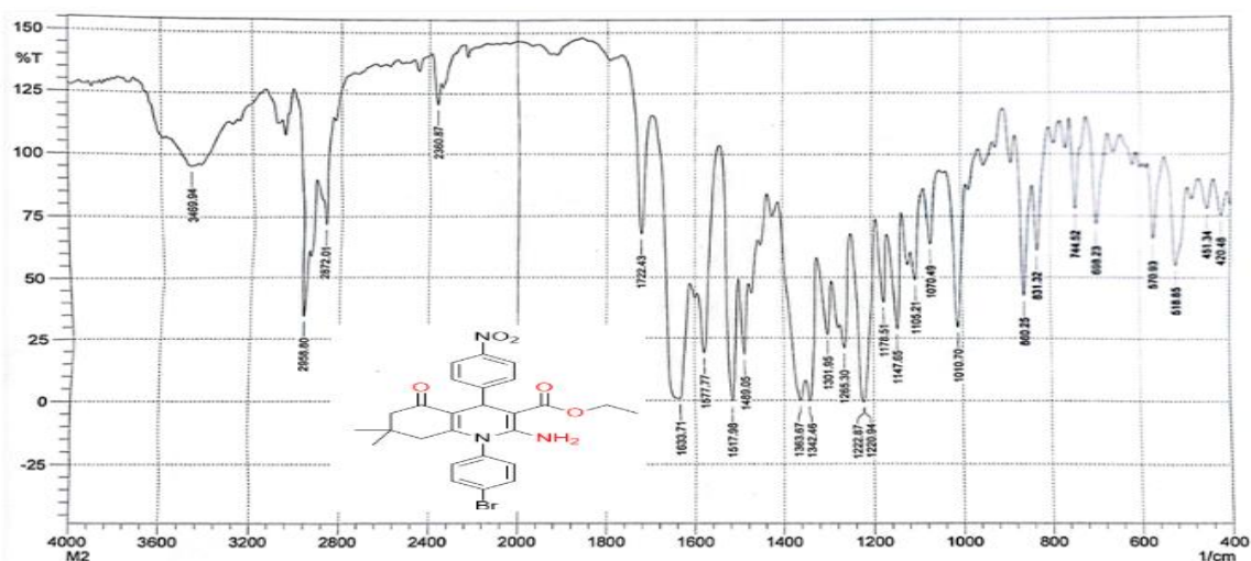
شكل (4) طيف IR للمركب BNO2
