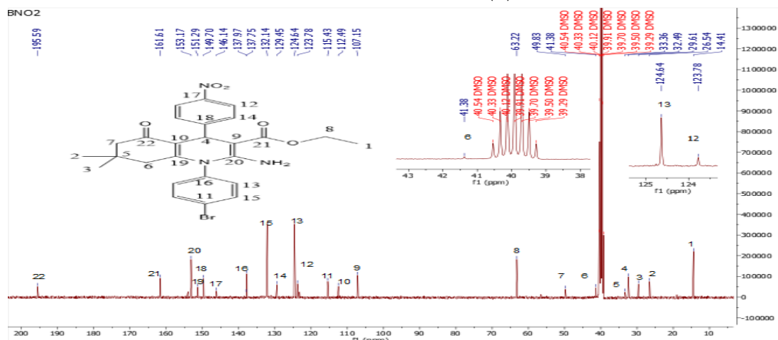
شكل (6) طيف C 13 NMR للمركب BNO2
