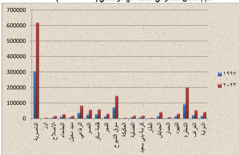
شكل (٤) حجم السكان الحضر في محافظة ذي قار لسنتي (١٩٩٧-٢٠٢٤)
