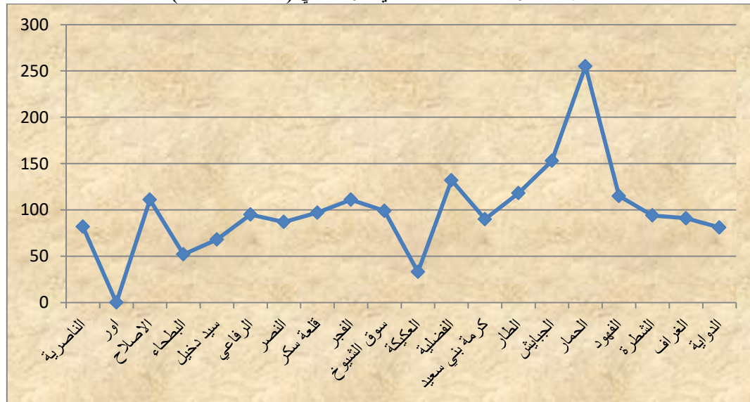
شكل (٣) نسبة التغير لسكان محافظة ذي قار لسنتي (١٩٩٧-٢٠٢٤)
