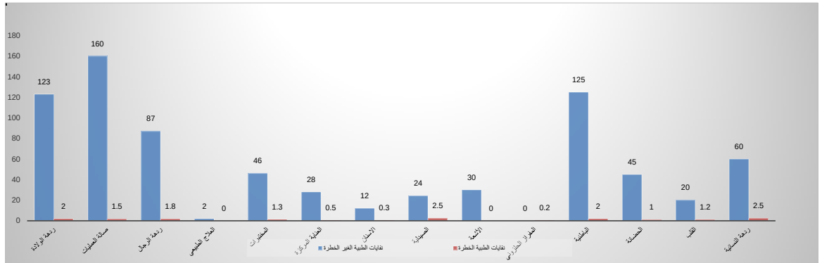
الشكل رقم (٦) يوضح كمية النفائات الطبية (كغم\اليوم) \ المصدر: بالاعتماد على جدول رقم (٥)
