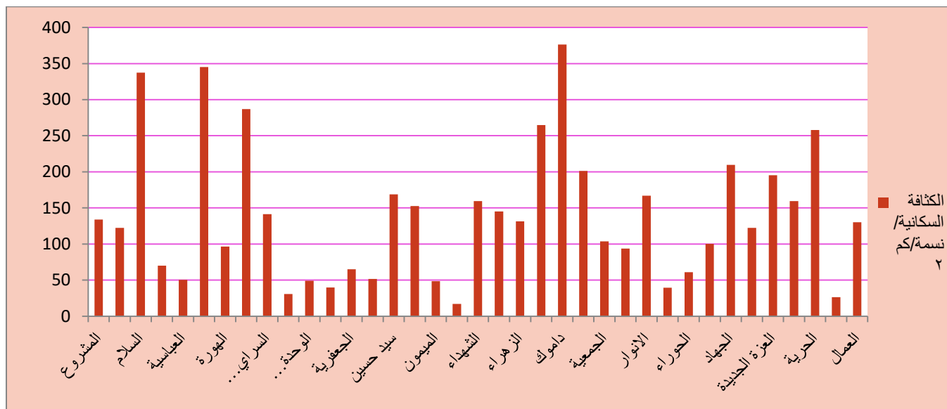
شكل (٣) التوزيع الكثافي لسكان مدينة الكوت بحسب الاحياء السكنية لعام ٢٠٢٤
