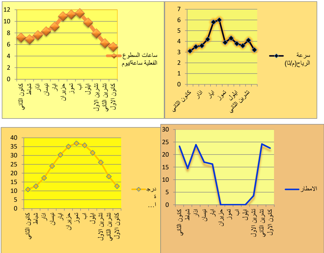
شكل (١) المعدلات الشهرية والسنوية لعناصر مناخ مدينة الكوت للمدة (٢٠١٤-٢٠٢٤)
