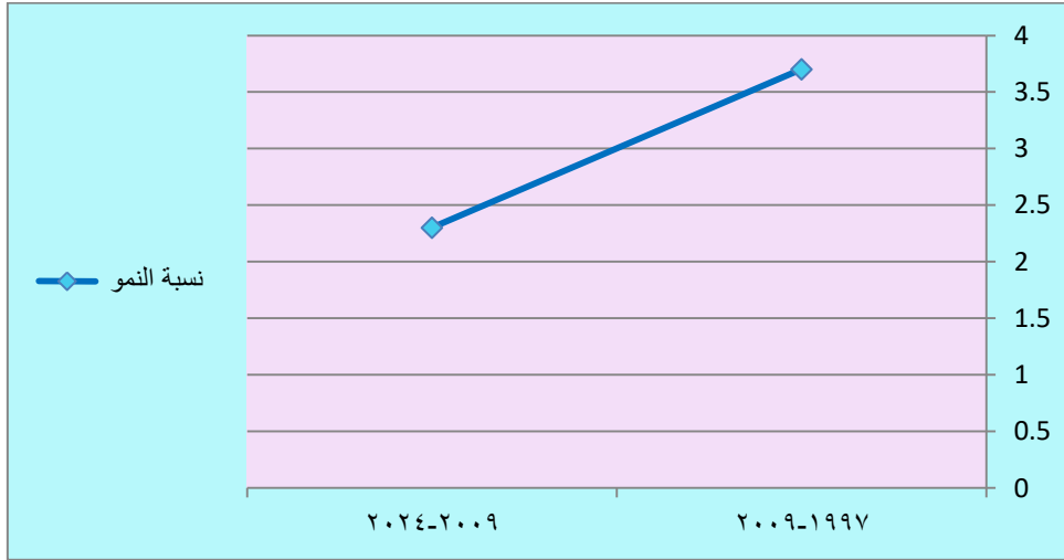
شكل (٢) نسبة النمو السكاني لمدينة الكوت للمدة (١٩٩٧-٢٠٢٤)
