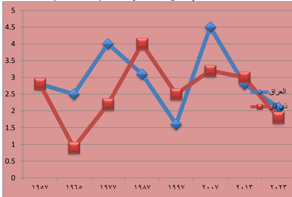
شكل (١) معدل النمو السكاني للعراق ومحافظة ذي قار للمدة (١٩٤٧-٢٠٢٤)
