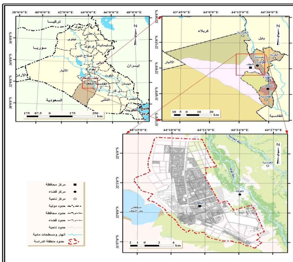
الشكل (٢): موقع منطقة الدراسة (مدينة النجف الأشرف) بالنسبة لمحافظة النجف والعراق،
