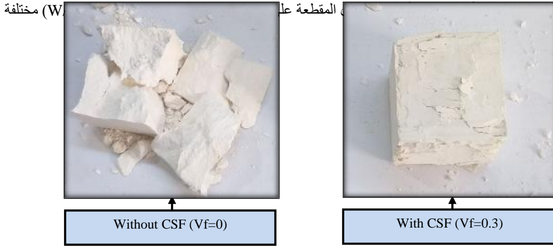
الشكل (٨): شكل العينات الفاشلة مع وبدون ألياف السيزال المقطعة
