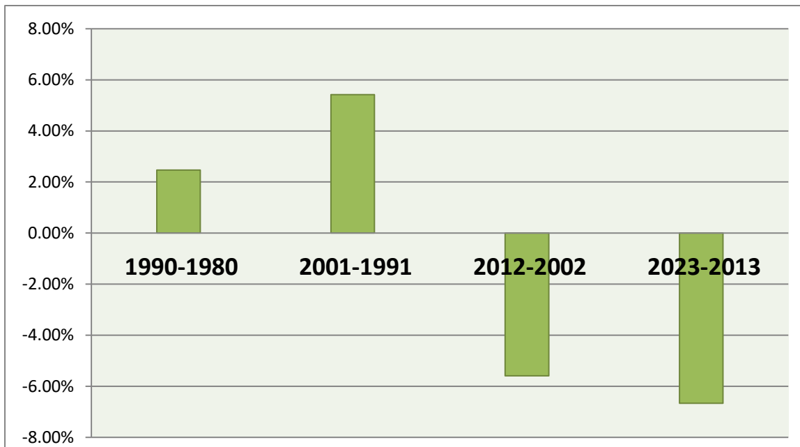
شكل (٢) معدل التغيير لكمية الامطار (ملم) خلال الفترات الاربعة في محافظة القادسية
