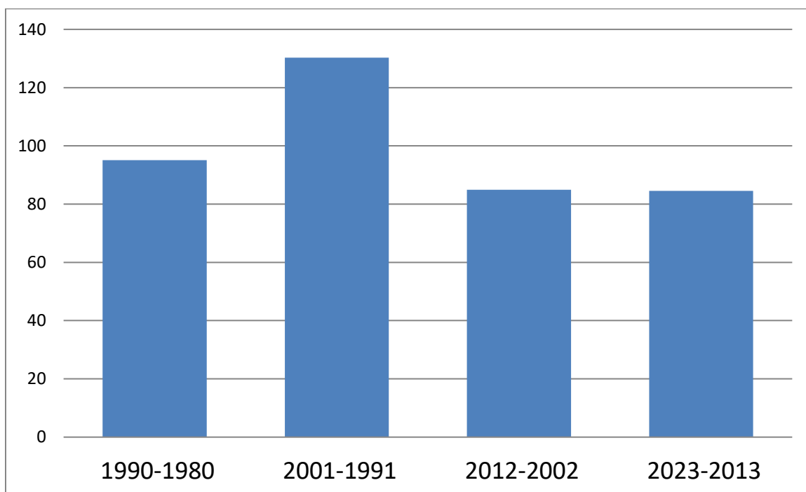
شكل (٤) متوسط سقوط الامطار (مم) خلال الفترات الاربعة في محافظة القادسية
