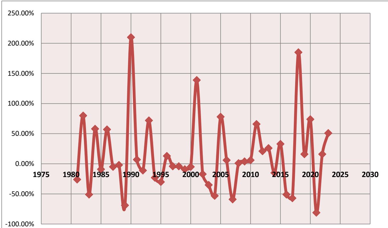
شكل (١) معدل التغير السنوي لكمية الامطار (مم) في محافظة القادسية
