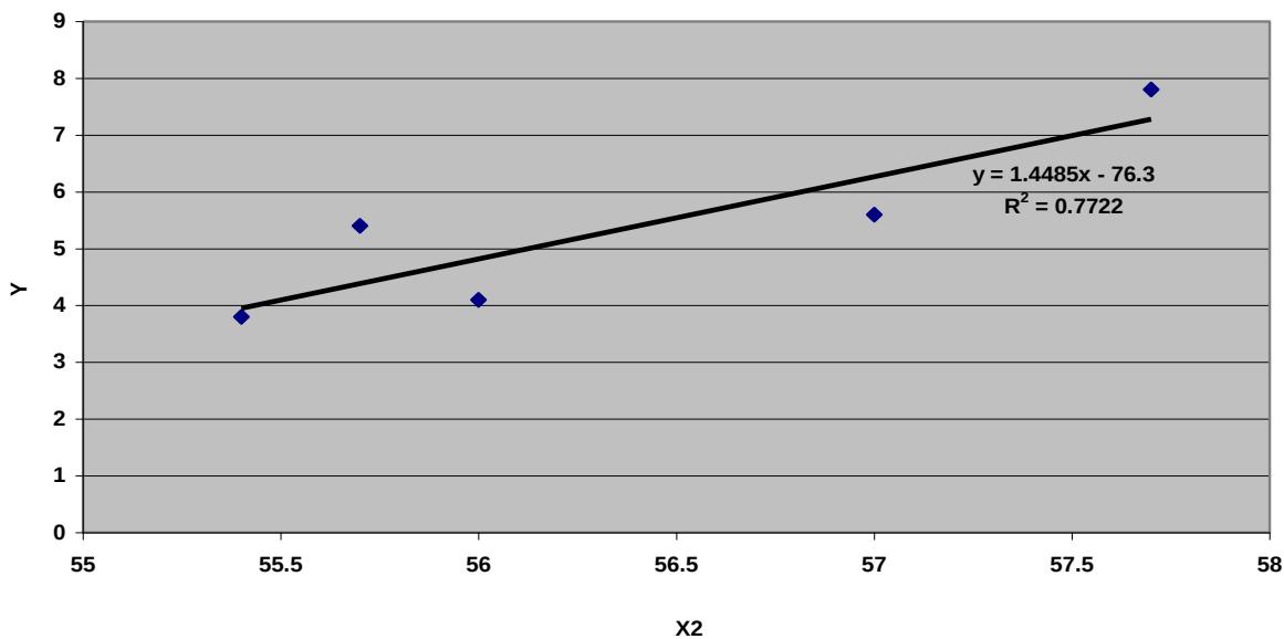
شكل (١) العلاقة بين معدل المجموع السنوي لعدد ايام حدوث العواصف الترابية والاشعاع الشمسي في محافظة الانبار.
