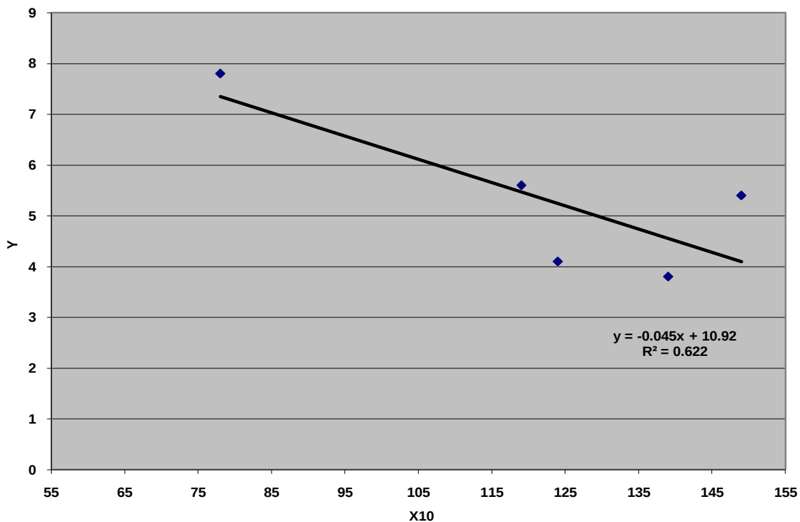
شكل (١٠) العلاقة بين معدل المجموع السنوي لعدد ايام حدوث العواصف الترابية وكمية الامطار في محافظة الانبار .
