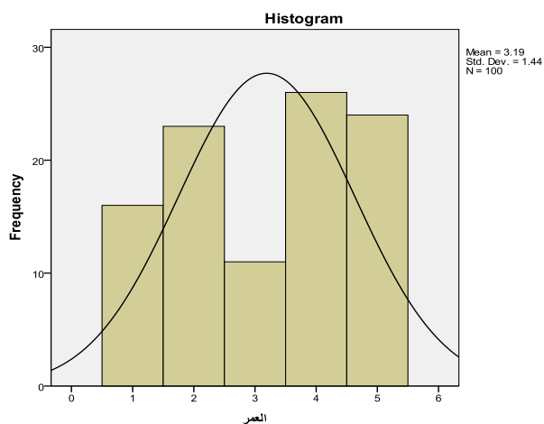
الشكل (١) العمر (X2) مقابل التكرارات
